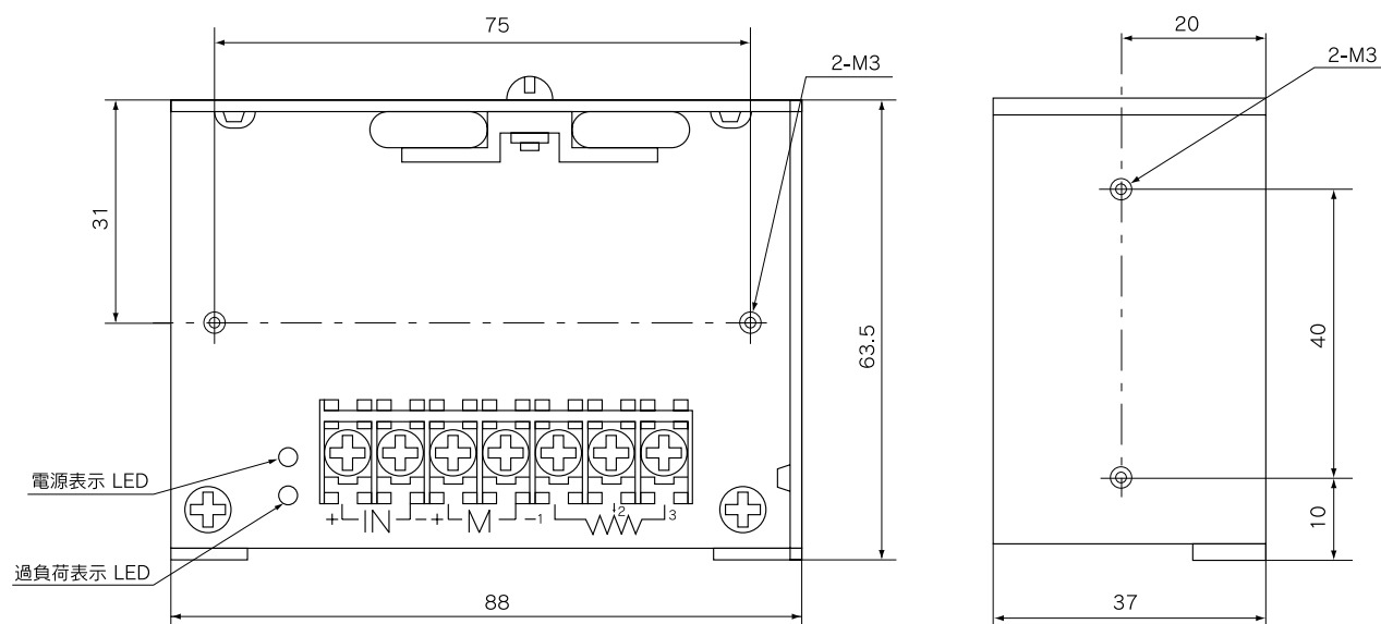
外形図
